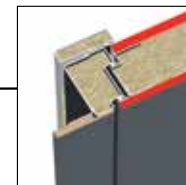
Накладки: зовнішня – МДФ 12 мм внутрішня – 12/16 мм
