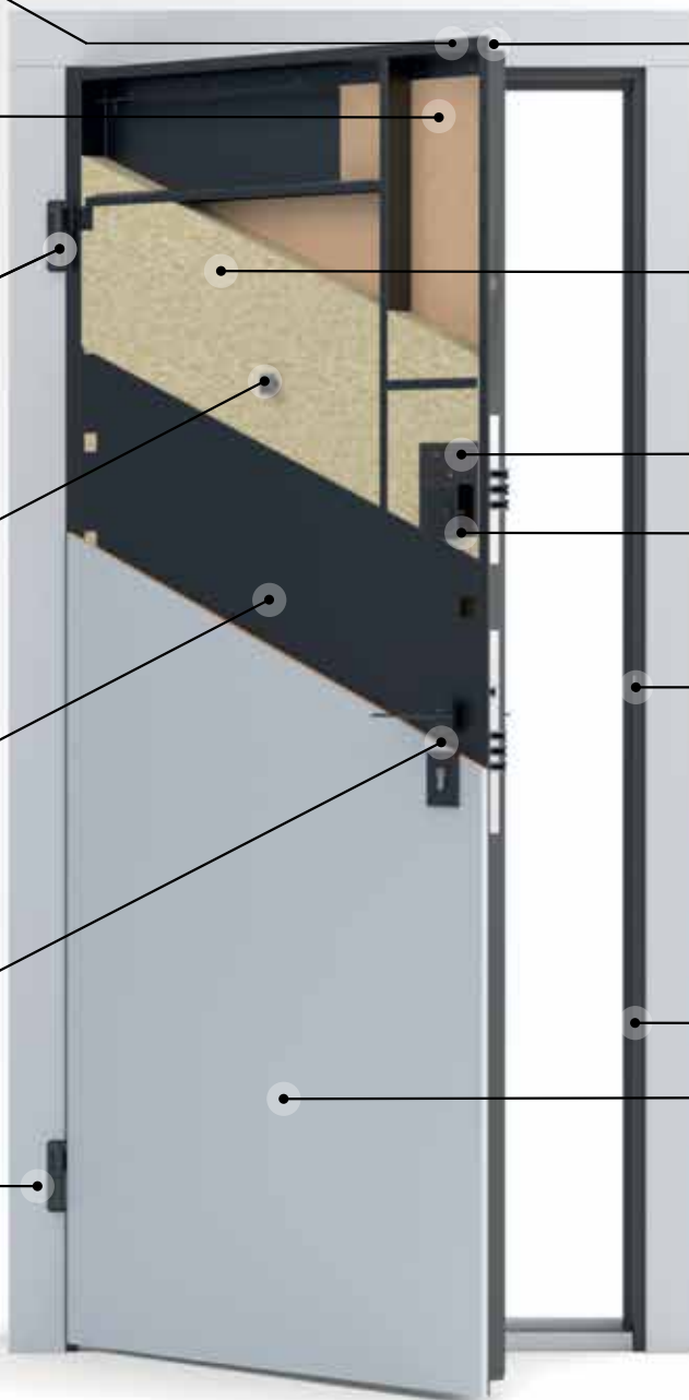
Ізоляція - базальтова вата 20 кг/м³ SWEETONDALE™
