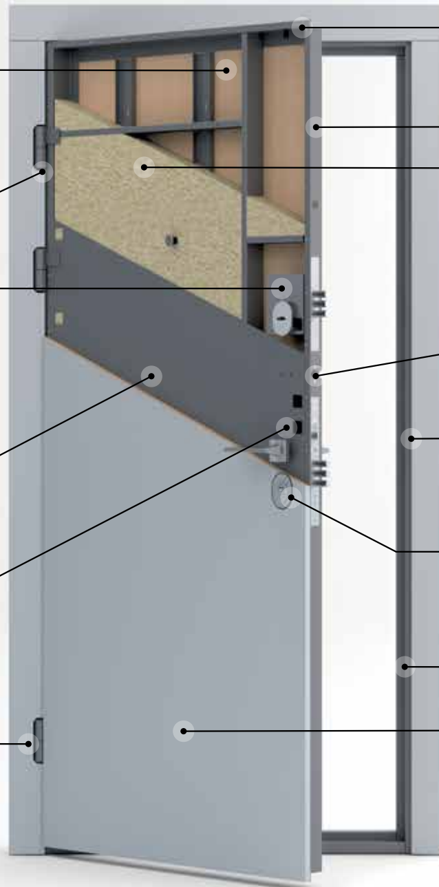
МДФ - 16 мм МДФ вологостійкий - 16 мм
