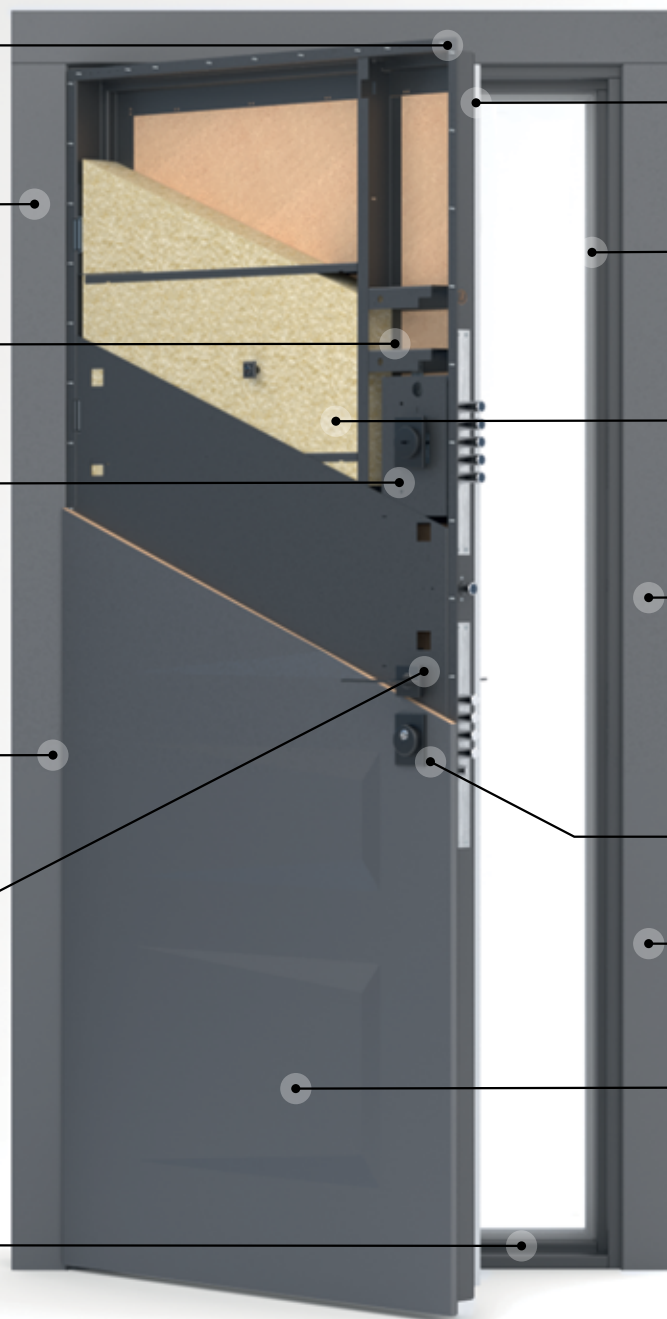
Терморозрив дверної коробки
